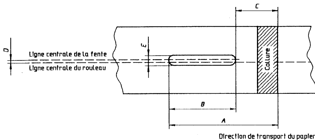
Figure 1 — Fente de détection de collure
