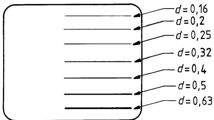
Figure 1 — Exemple de réalisation d'indicateur de qualité d'image à fils
