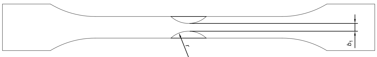
Figure 2 — Éprouvette destinée au mesurage de la résistance à la fissuration dans un environnement donné sous contrainte de traction, préparée par usinage de l'éprouvette afin d'obtenir un rétrécissement central identique à celui de la petite éprouvette de traction (voir Figure 1 )
