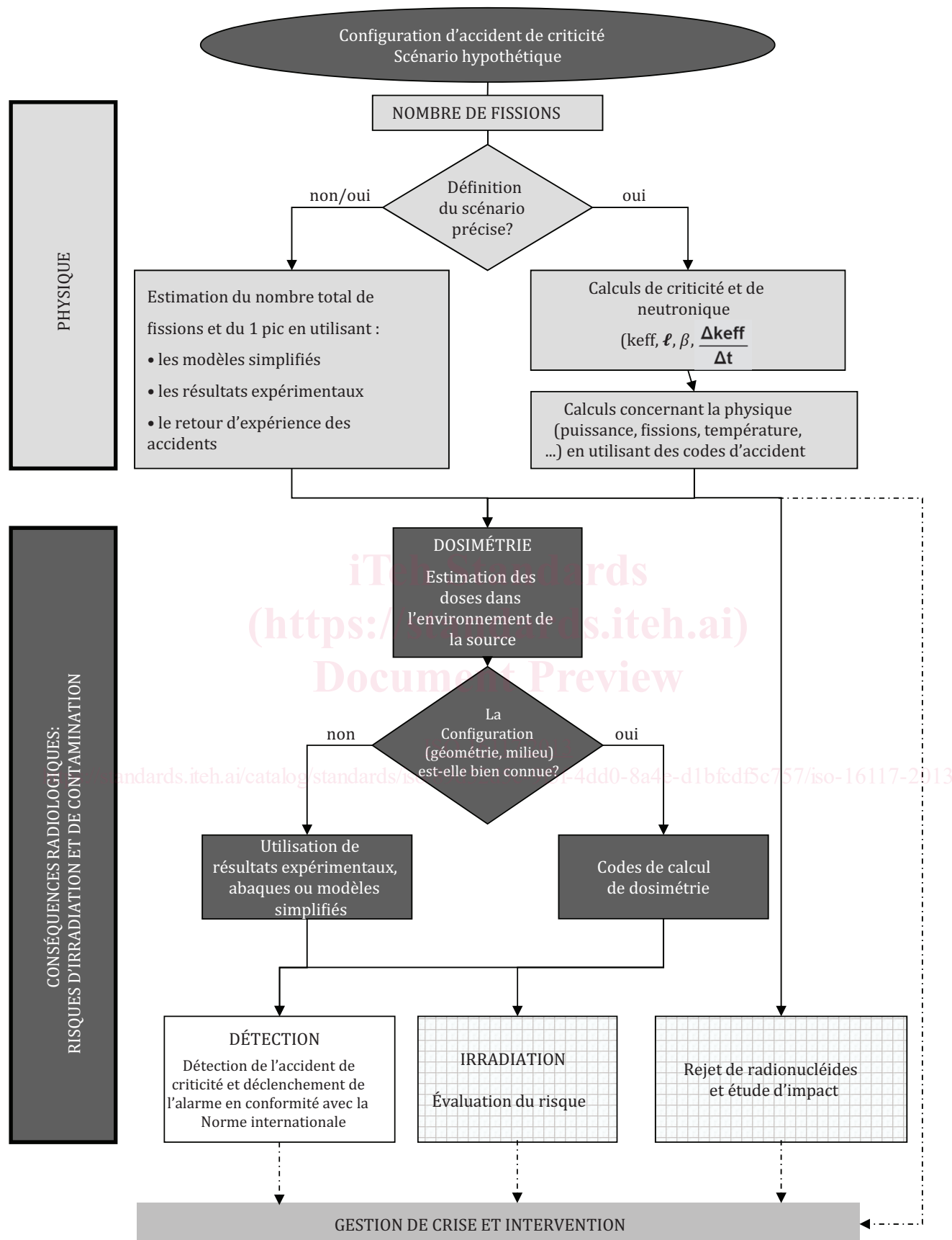
Figure A.1 — Schéma fonctionnel d'une analyse d'un accident de criticité
