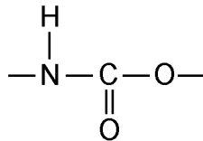
Figure A.1 — Groupe uréthane
