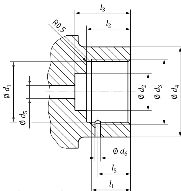
Figure 4 — Sortie de robinet pour pression de 232 bar
