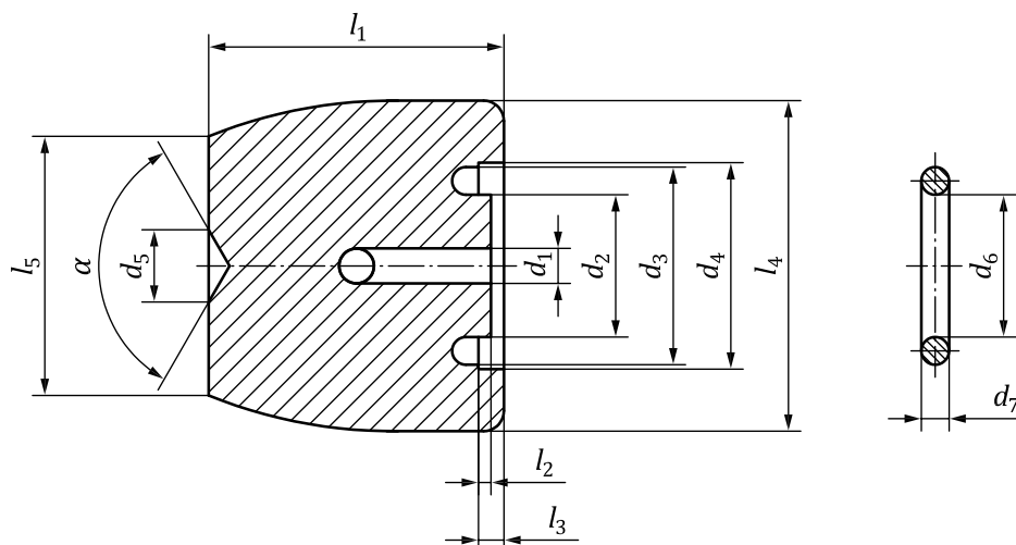
Figure 2 — Dimensions de sortie du robinet
