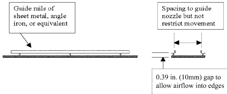
FIG. 1 Guide Rails
