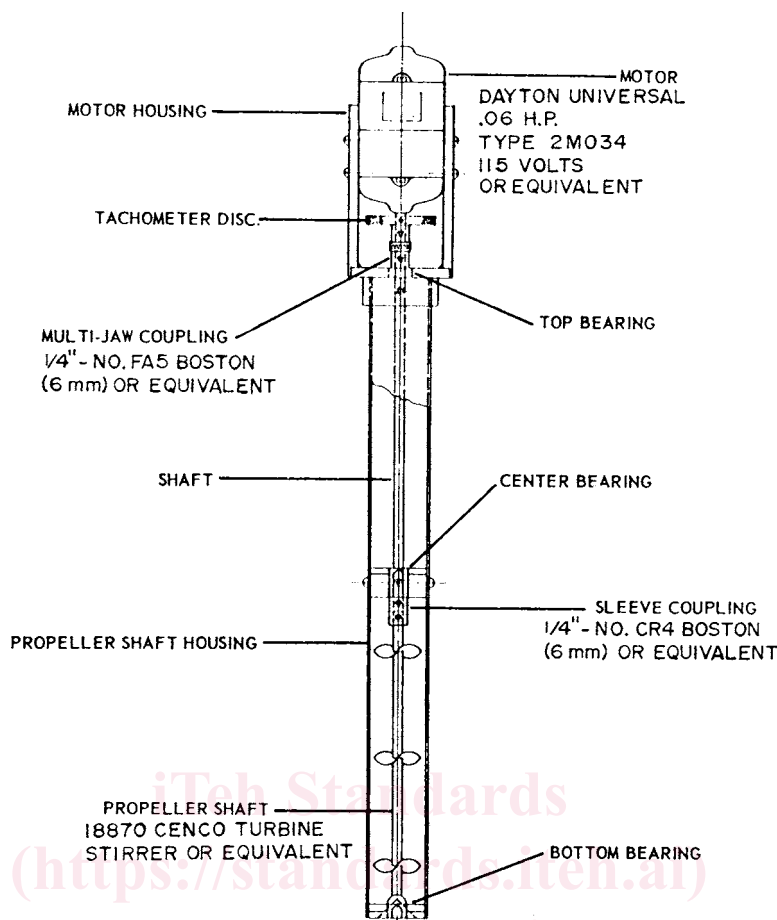
FIG. 1 Stirrer
