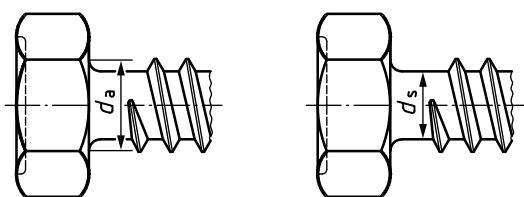
Figure 4 — Diamètre intérieur de la face d'appui, d_a , et diamètre de tige, d_s
