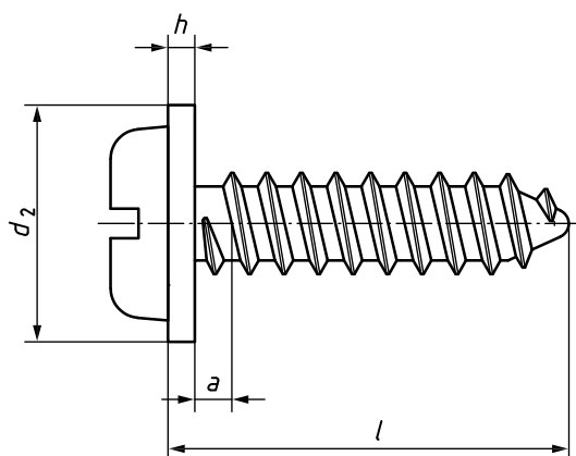
Figure 3 — Vis à tôle à tête cylindrique bombée plate fendue, par exemple à bout arrondi (type R)
