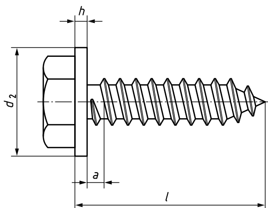
Figure 1 — Vis à tôle à tête hexagonale, par exemple à bout pointu (type C)
