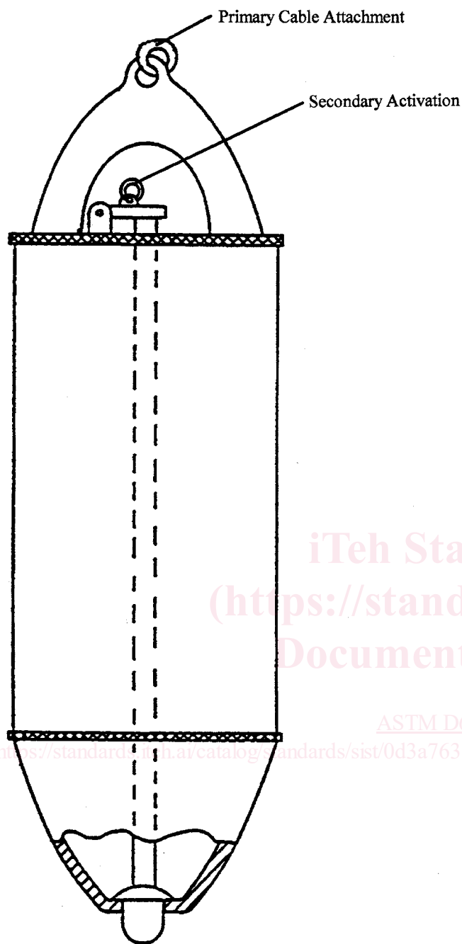
FIG. 4 Bacon Bomb
