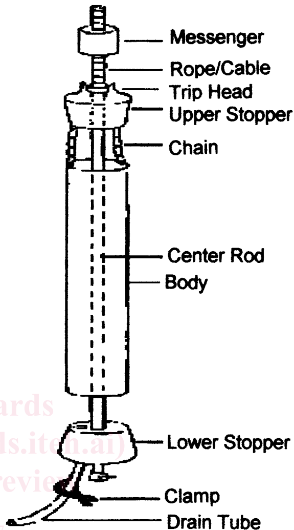
FIG. 6 Kemmerer Sampler
