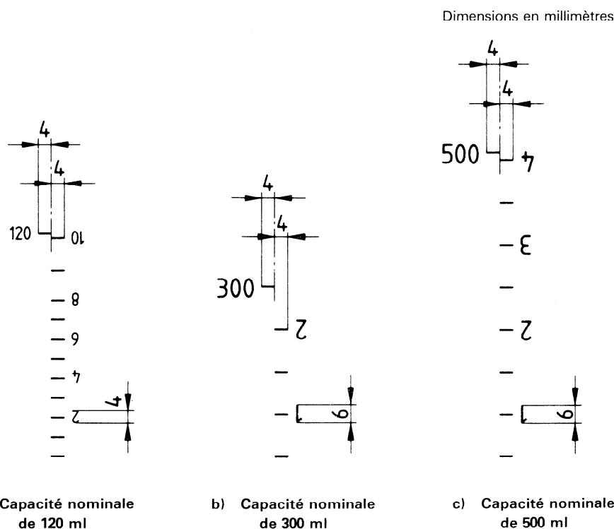
Figure 3 — Graduations pour flacons de transfusion ayant un diamètre d'ouverture nominal du col 22,5 mm
