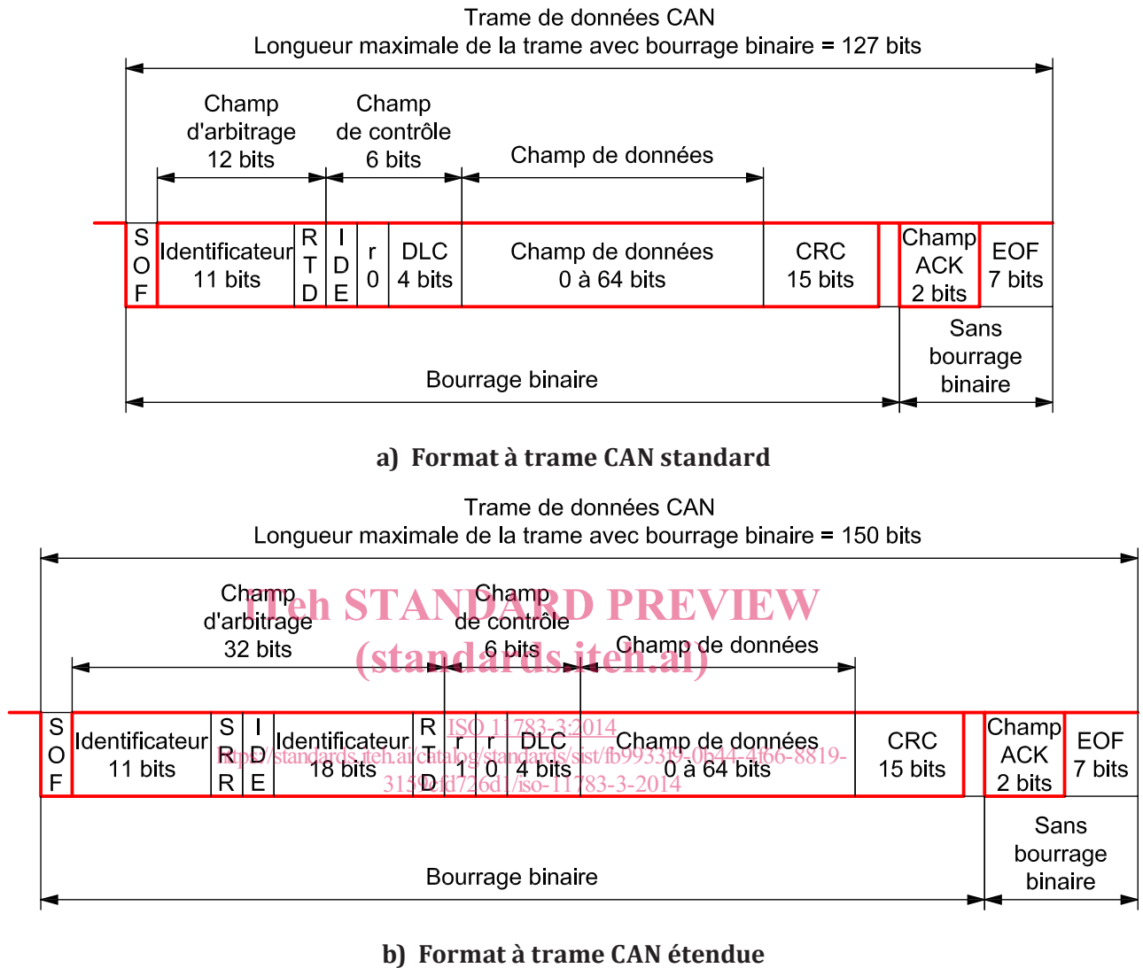
Figure 1 — Trames de données CAN
