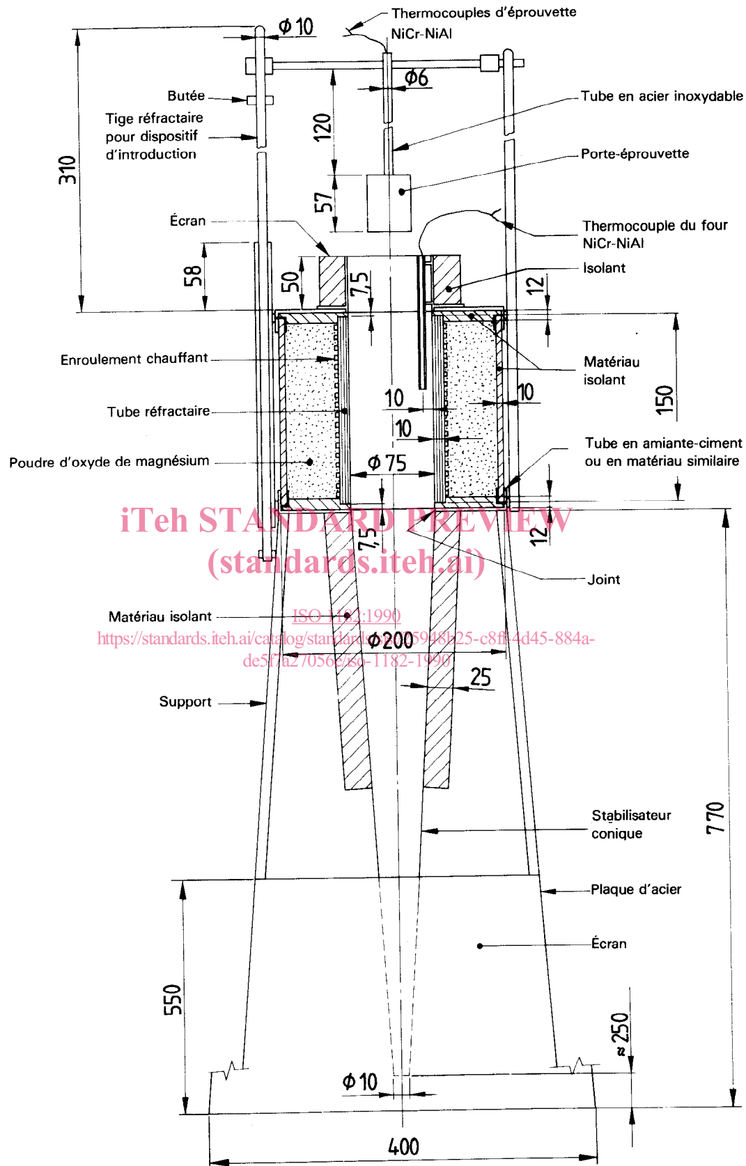
Figure 1 — Disposition générale de l'appareillage d'essai
