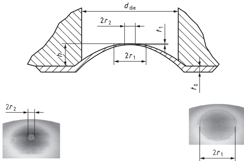
Figure 4 — Choix de r_1 et r_2 pour le calcul de la contrainte vraie et de la déformation vraie pour chaque stade de formage
