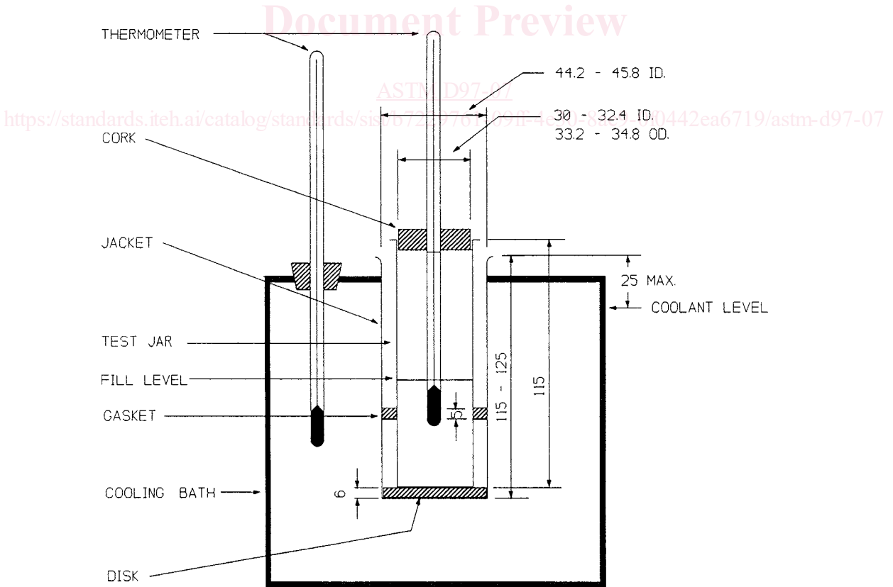
FIG. 1 Apparatus for Pour Point Test
