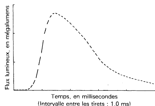
Figure 2 — Flux lumineux en fonction du temps
