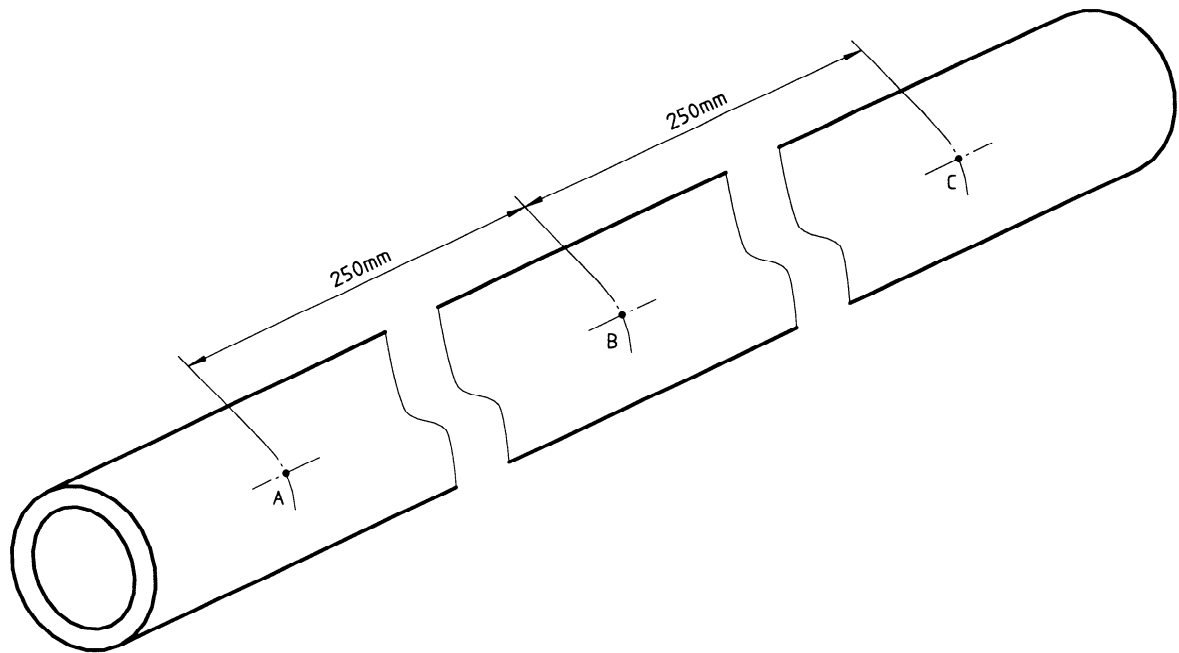
Figure 1 — Mesurage de la stabilité dimensionnelle
