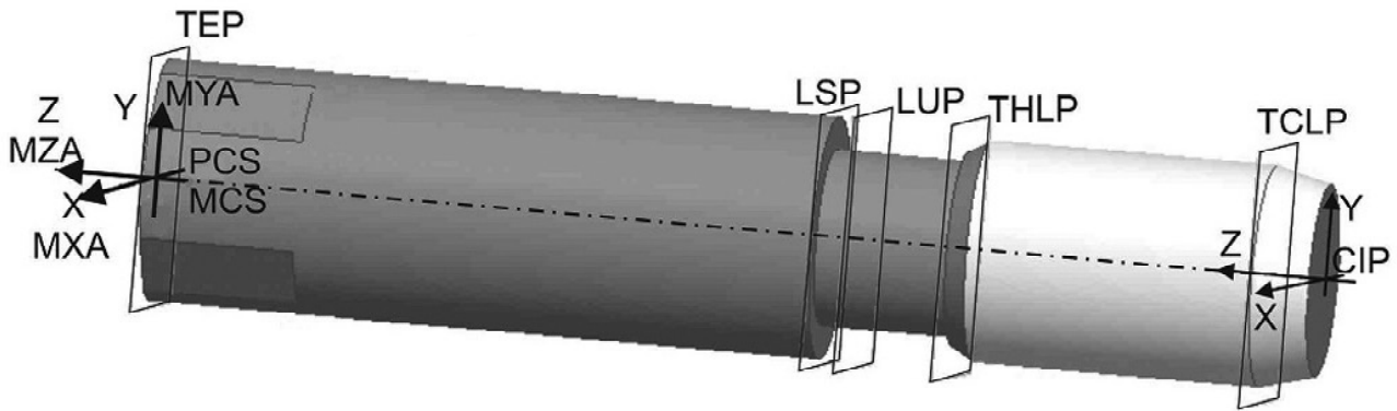
Figure 3 — Orientation du MCS et du PCS, système de référence (exemple)
