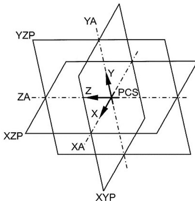
Figure 1 — Système de référence
