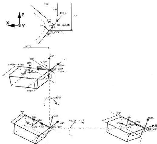
Figure 6 — Angle de coupe axial et radial sur une plaquette
