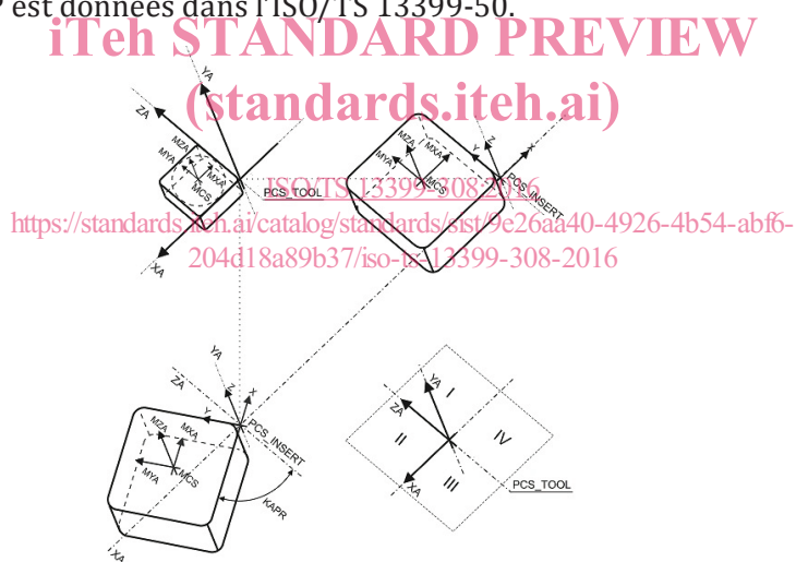
Figure 5 — Orientation du PCS_INSERT, du MCS_INSERT et du PCS_TOOL sur l'angle de direction d'arête en bout
