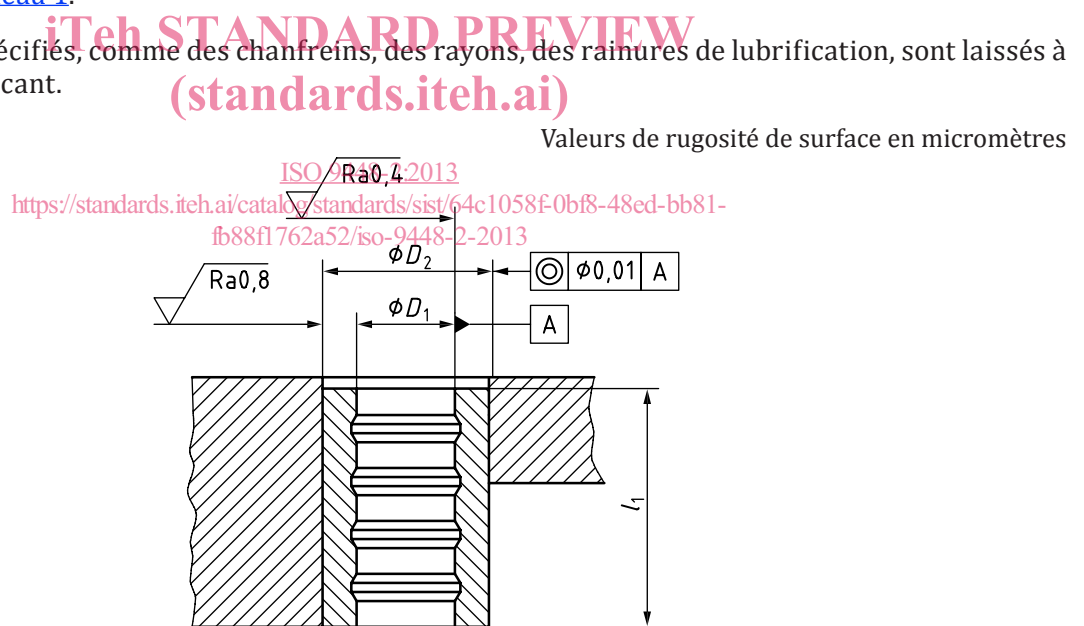
Figure 1 — Forme A, bagues lisses pour guidage lisse, type 1
