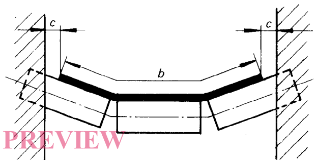
FIGURE 1 — Rouleaux porteurs
