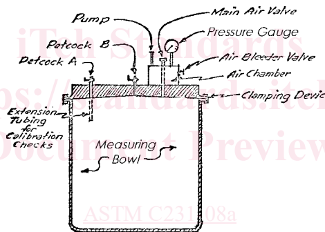
FIG. 2 Schematic Diagram—Type-B Meter
