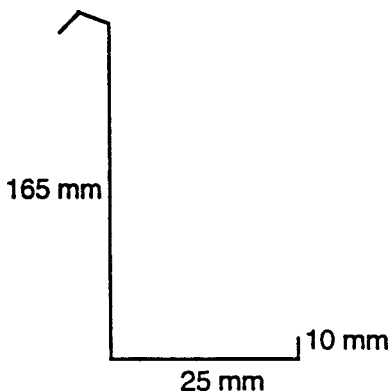
FIG. 1 Wire Hanger
