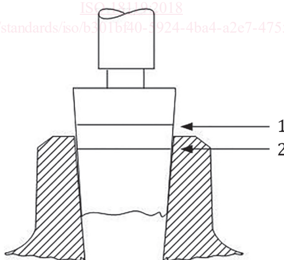
Figure 1 — Exemple de tampon lisse de contrôle étalonné pour contrôler le haut du filetage (filetage non conforme)
