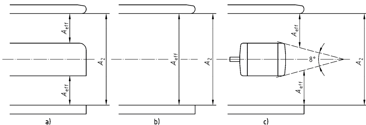
Figure 1 — Aires effective et brute de refoulement du ventilateur
