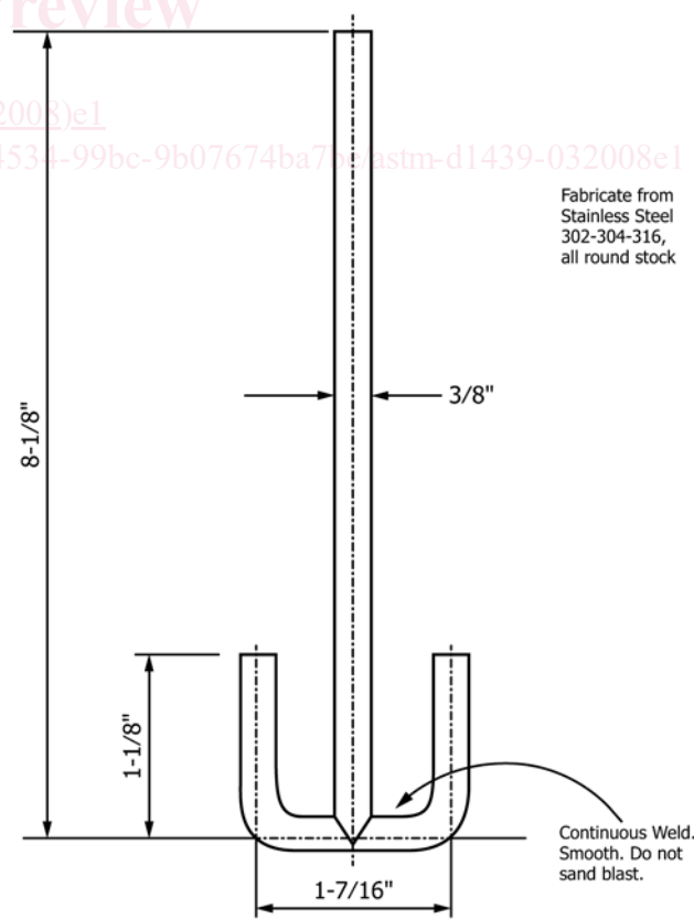
FIG. 1 Stirrer
