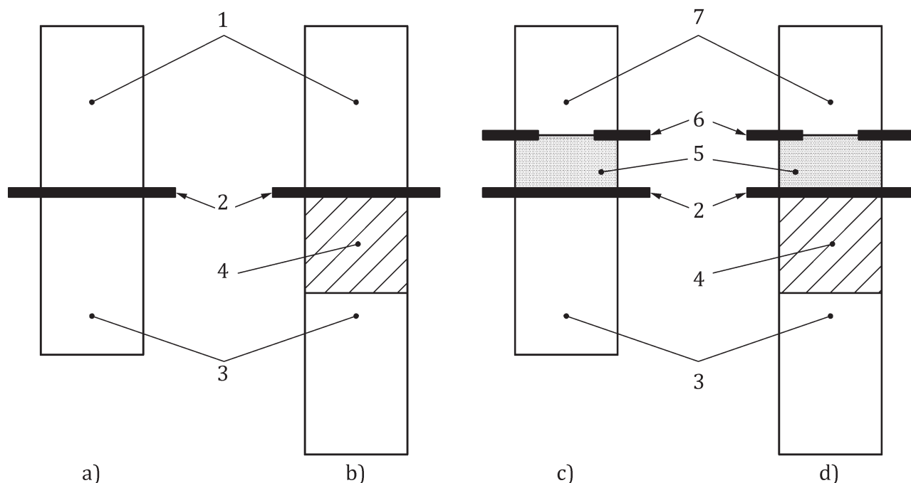
a) Interface directe b) Interface avec support intermédiaire c) Interface directe (en cas de combinaison d'un actionneur multitour et d'un réducteur) d) Interface avec support intermédiaire (en cas de combinaison d'un actionneur multitour et d'un réducteur)
