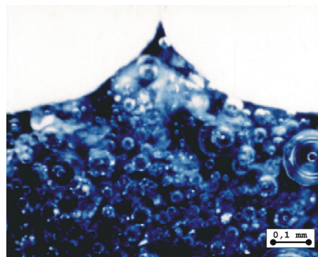
a) Émail de couverture blanc avec lignes de tension détectables au niveau macroscopique b) Vue latérale, émail de couverture blanc laissant apparaître l'émail de masse sombre
