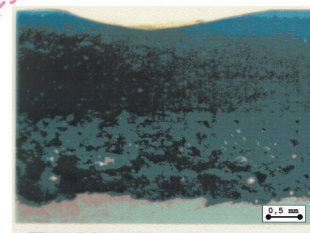
c) Revêtement d'émail exempt de défauts sous craquelure de séchage
