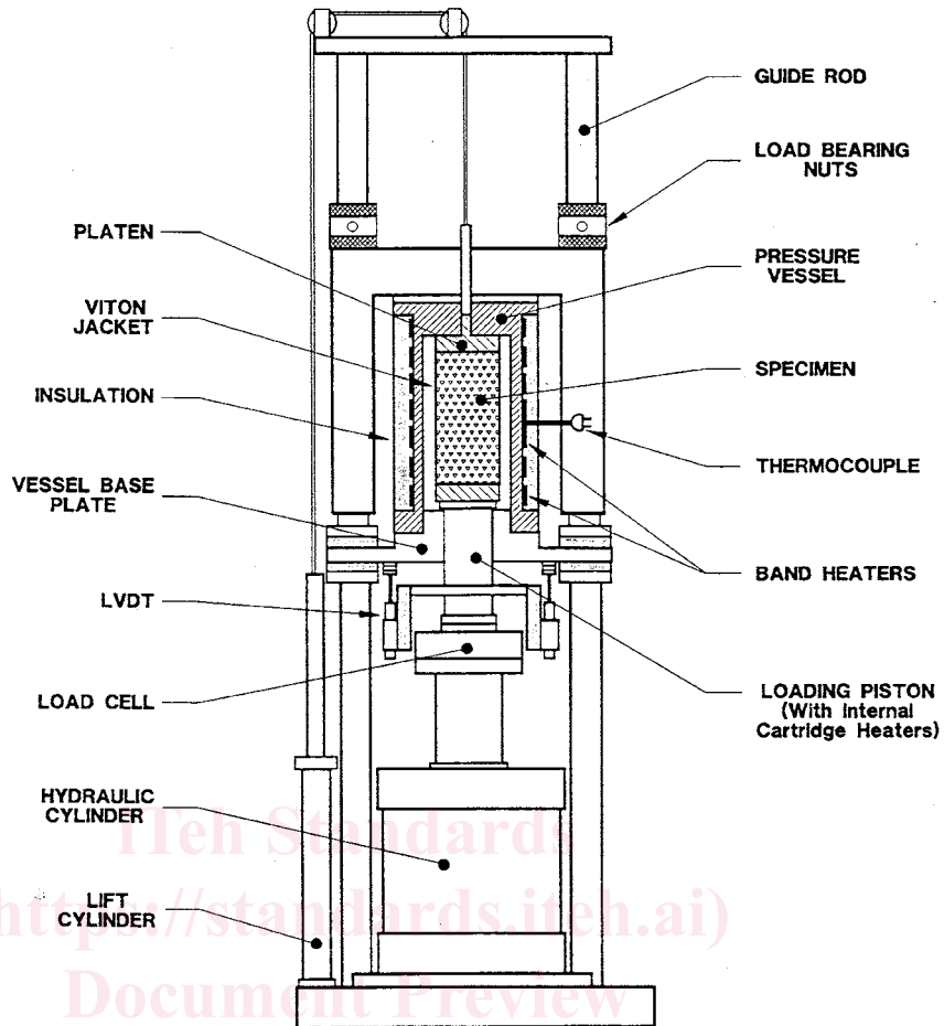
FIG. 1 Test Apparatus
