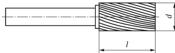
Figure 1 — Fraises-limes en métaux durs, forme A
