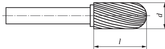
Figure 1 — Fraises-limes en métaux durs, forme C
