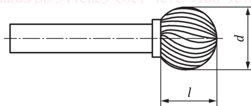
Figure 1 — Fraises-limes en métaux durs, forme D
