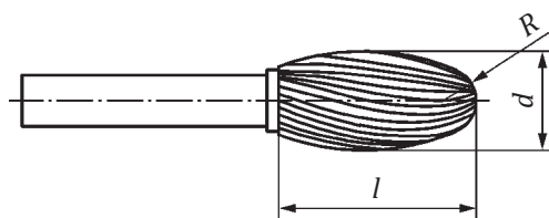
Figure 1 — Fraises-limes en métaux durs, forme E
