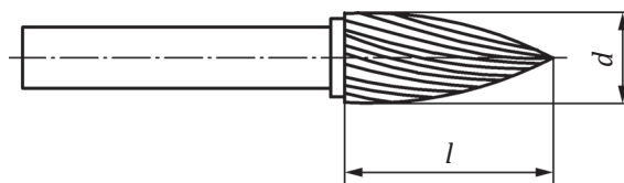
Figure 1 — Fraises-limes en métaux durs, forme G
