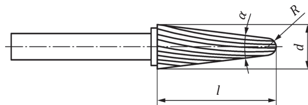
Figure 1 — Fraises-limes en métaux durs, forme L
