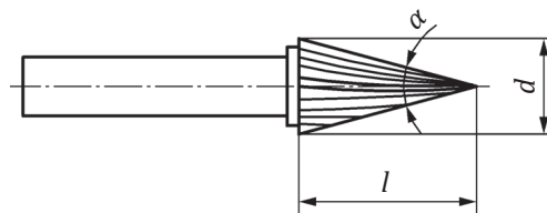
Figure 1 — Fraises-limes en métaux durs, forme M
