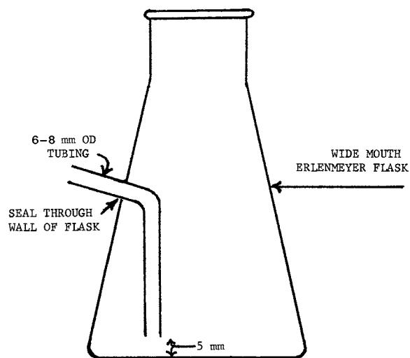
FIG. 1 Titration Flask
