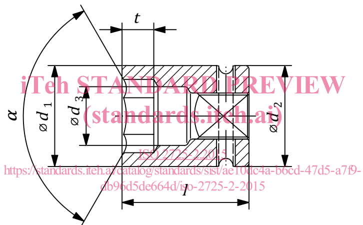
Figure 1 — Douilles avec d_1 < d_2
