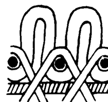
Représentation de deux boucles successives d'un velours
