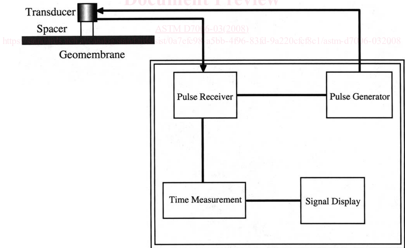
FIG. 1 Test Apparatus
