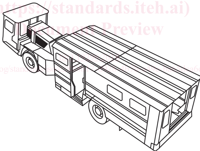
Figure 7 — Transporteur de personnel
