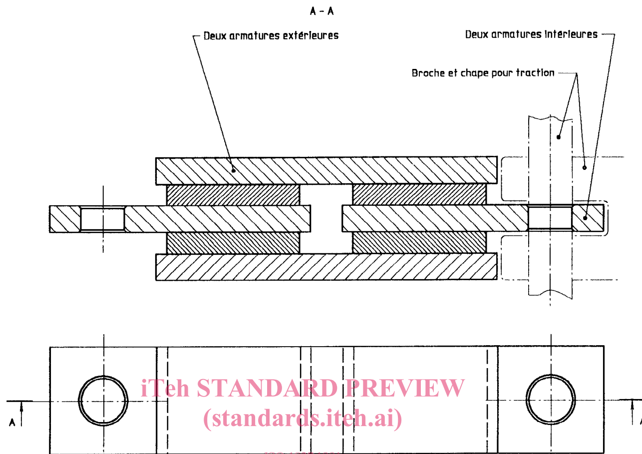
Figure 1 — Dispositions de l'éprouvette
