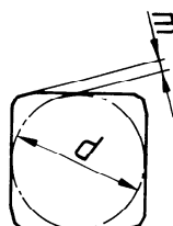
Cas 3 — Plaquettes avec arêtes de planage (voir note 1 du tableau 9)
