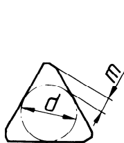
Cas 3 — Plaquettes avec arêtes de planage (voir note 1 du tableau 9)
