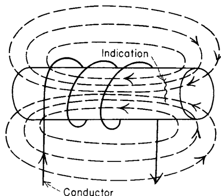
FIG. 1 Longitudinal Magnetization
