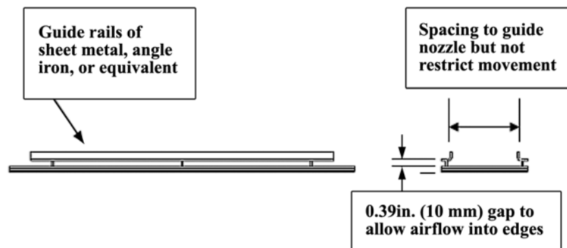
FIG. 1 Guide Rails
