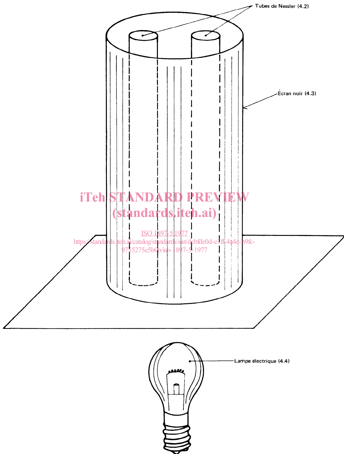
FIGURE – Appareillage pour l'évaluation des matières insolubles dans l'eau
