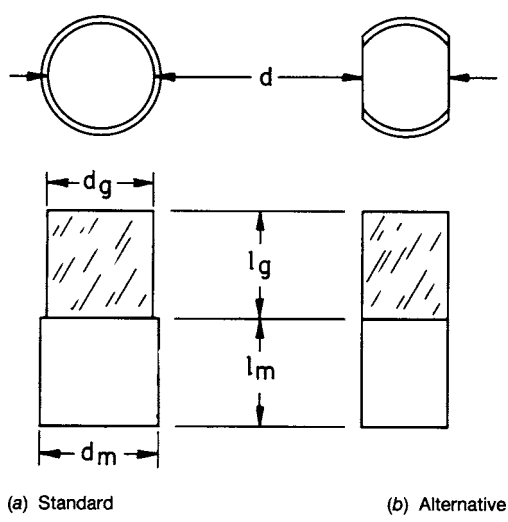
FIG. 1 Rod Seals
