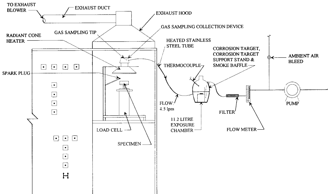
FIG. 1 Cone Corrosimeter
