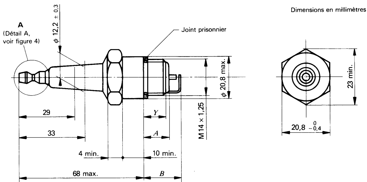
Figure 1 — Bougie d'allumage M 14 × 1,25 à siège plat
