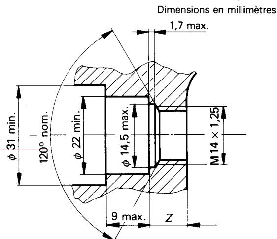
Figure 3 — Autre configuration admise du logement dans la culasse
