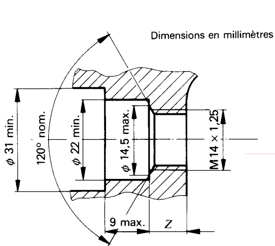
Figure 2 — Logement de la bougie dans la culasse
