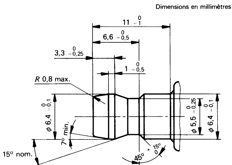
Figure 4 — Borne monobloc (détail A de la figure 1)
