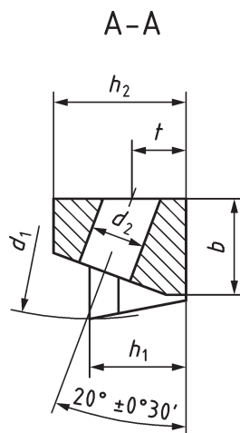
Figure 4 — Section A-A pour les cartouches ayant une hauteur h_1 = 6 \text{ mm} , 8 \text{ mm} , 10 \text{ mm} ou 12 \text{ mm}
