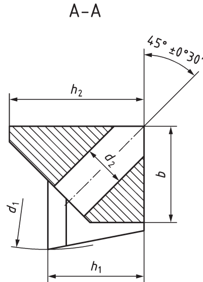
Figure 5 — Section A-A pour les cartouches ayant une hauteur h_1 = 16 mm, 20 mm ou 25 mm
