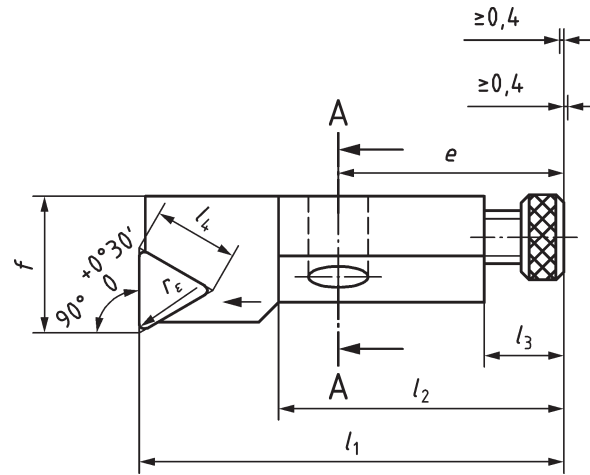
Figure 2 — Forme F ayant une hauteur h_1 = 8 \text{ mm} , 10 \text{ mm} , 12 \text{ mm} , 16 \text{ mm} et 20 \text{ mm} avec plaquette triangulaire
